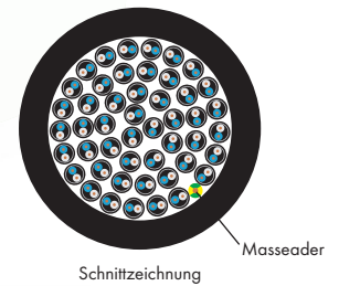
Schnittzeichnung
