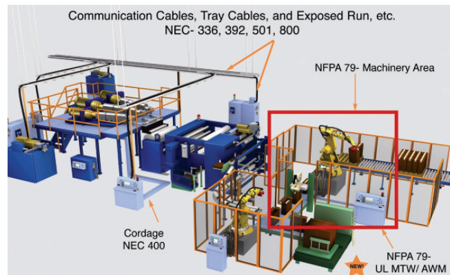
Das Schema einer industriellen Maschine zeigt wesentliche Anwendungen von Kabel und Leitungen mit Verweis auf die zugehörigen Abschnitte in NEC®/NFPA. ‚NEC®‘ ist ein Markenzeichen der National Fire Protection Association <NFPA>.
