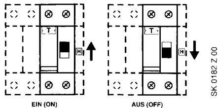
Abb. 6 Schaltstellungen
