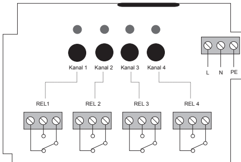
Bild 1: Anschlussschema und Bedienelemente
