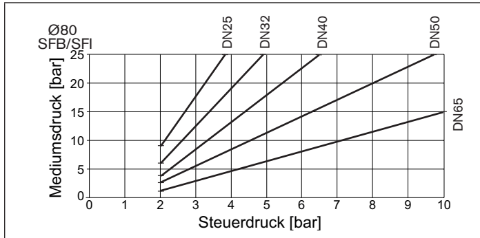
Bild 16: Druckdiagramm, Antrieb ø 80 mm, Steuerfunktion B und I, Anströmung unter Sitz
