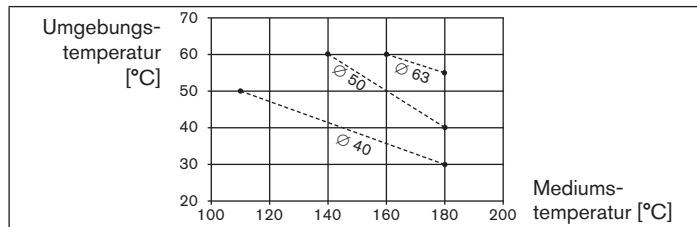
Bild 5: Temperaturbereich der maximalen Mediums- und Umgebungstemperatur bei PA Antrieben
