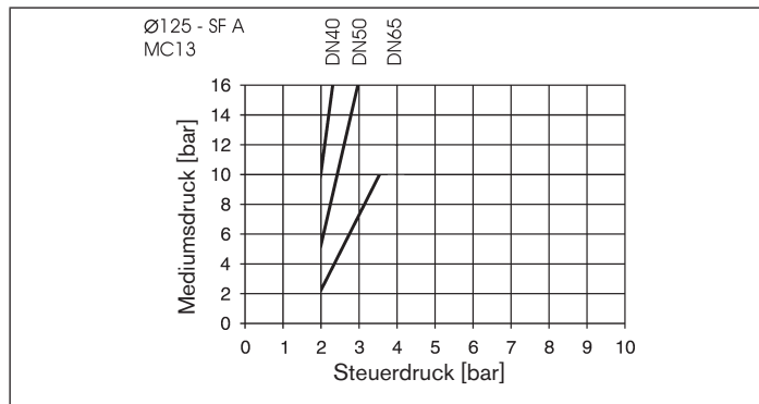
Bild 14: Druckdiagramm, Antrieb ø 125 mm, Steuerfunktion A, Anströmung über Sitz
