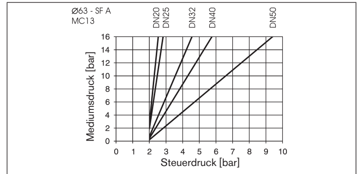
Bild 11: Druckdiagramm, Antrieb ø 63 mm, Steuerfunktion A, Anströmung über Sitz
