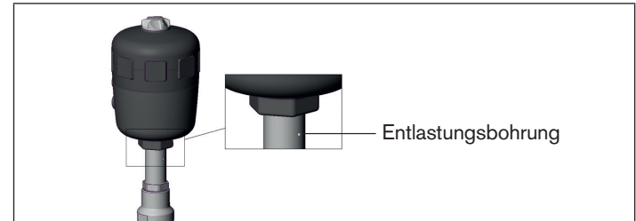
Bild 21: Entlastungsbohrung
