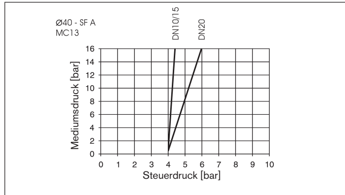
Bild 9: Druckdiagramm, Antrieb ø 40 mm, Steuerfunktion A, Anströmung über Sitz
