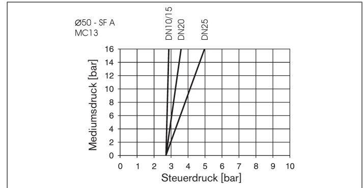
Bild 10: Druckdiagramm, Antrieb ø 50 mm, Steuerfunktion A, Anströmung über Sitz
