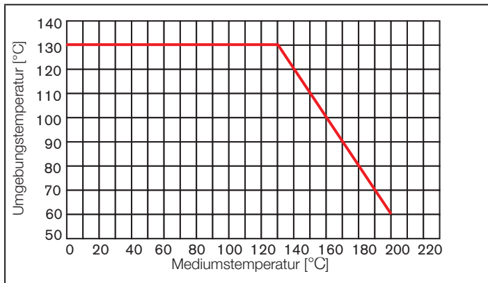
Bild 6: Derating CLASSIC ANTG40
