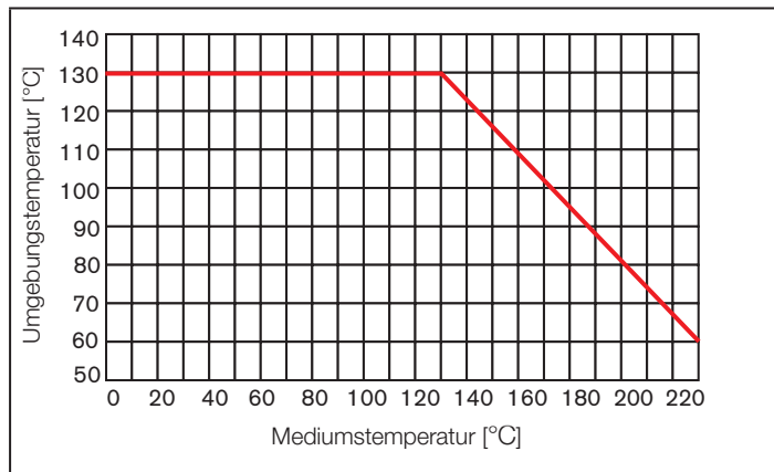
Bild 7: Derating CLASSIC ANTG50, 63, 80
