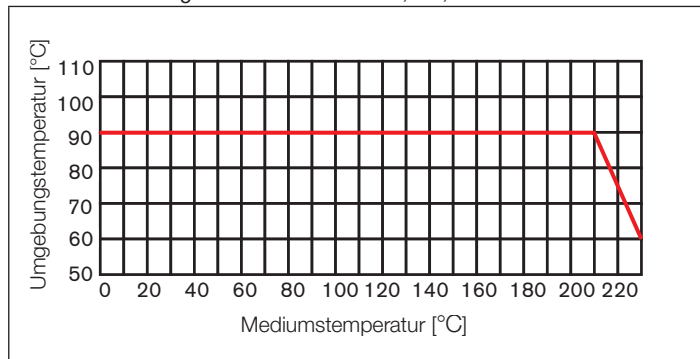
Bild 8: Derating CLASSIC ANTG100, 125
