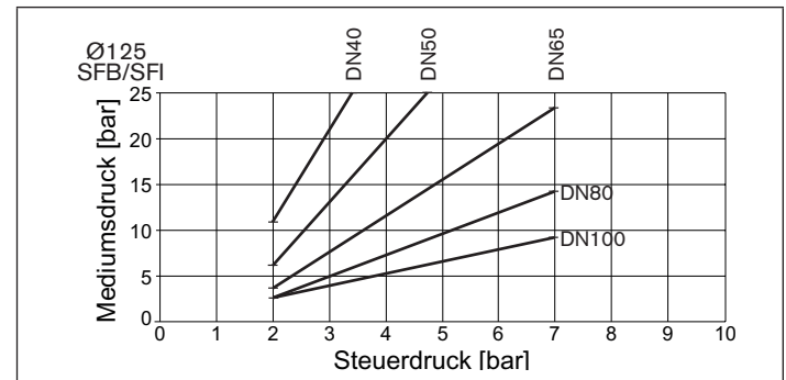
Bild 18: Druckdiagramm, Antrieb ø 125 mm, Steuerfunktion B und I, Anströmung unter Sitz
