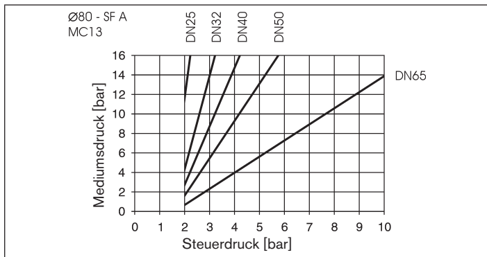
Bild 12: Druckdiagramm, Antrieb ø 80 mm, Steuerfunktion A, Anströmung über Sitz
