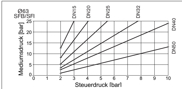
Bild 15: Druckdiagramm, Antrieb ø 63 mm, Steuerfunktion B und I, Anströmung unter Sitz
