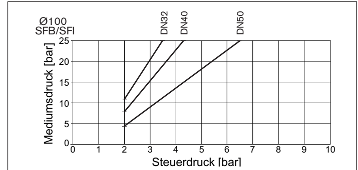
Bild 17: Druckdiagramm, Antrieb ø 100 mm, Steuerfunktion B und I, Anströmung unter Sitz
