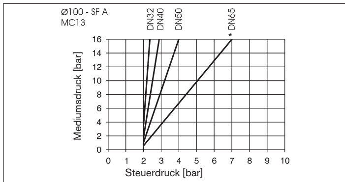
Bild 13: Druckdiagramm, Antrieb ø 100 mm, Steuerfunktion A, Anströmung über Sitz
