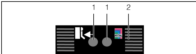
Abb. 8: Frontseite des Zugangssensors
