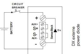
Batterielader-Modus (Fig.7)
