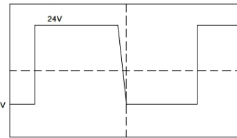
Schneller Spannungsabbau mit Stromsenke
