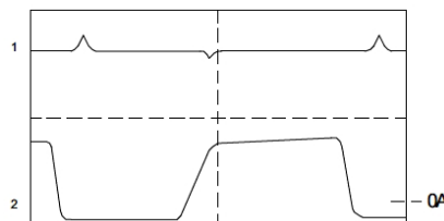
Dynamisches Lastverhalten mit PSINK: Laststrom wechselt zwischen positive und negativ
