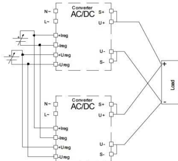
Parallelschaltung (Fig.2)
