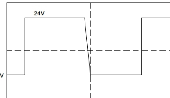
Schneller Spannungsabbau mit PSINK
