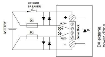
Senseanschluss absichern (Fig.8)
