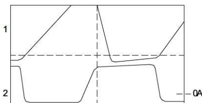
Dynamische Lastreaktion ohne PSINK: negativer Laststrom durch Rückespeisung entsteht
