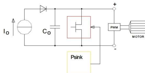
Mit PSINK Bremsenergie wird absorbiert
