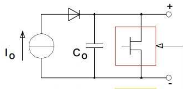
Abb.7 Netzteil mit PSINK
