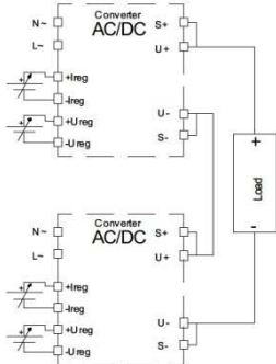
Serienschaltung (Fig.1)
