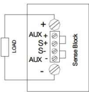
Lokales Sensing (Fig.5)
