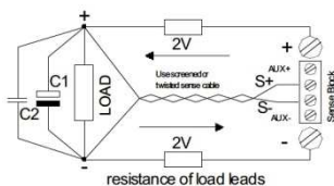
Maximal mögliche Kompensation (Fig.9)
