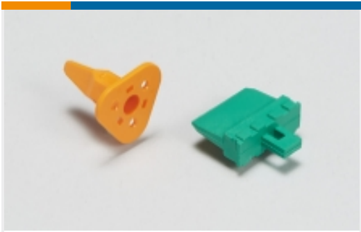
Verriegelung und Positionssicherung für Kfz-Steckverbinder(15)
