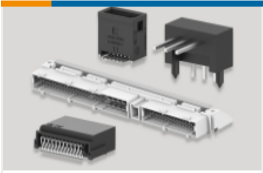
Leiterplatten-Stift- und Buchsenleisten (40)
