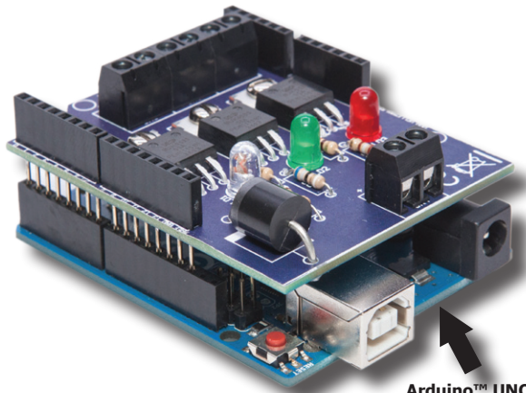
Arduino™ UNO (nicht mitgeliefert)
