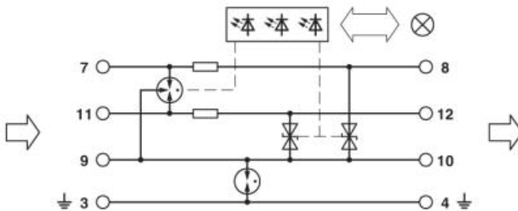
Schaltplan
