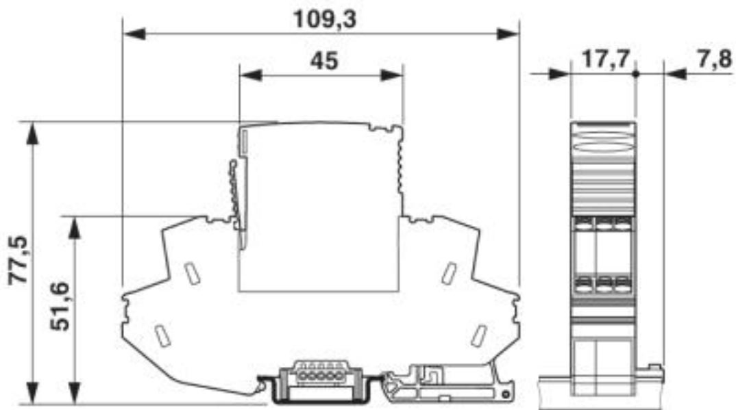
Maßzeichnung
