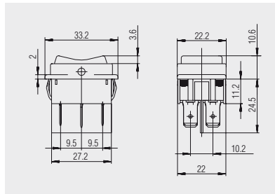
Steckanschluss 6.3 Grundtyp 1839
