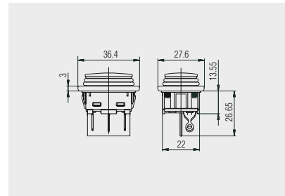
Lötanschluss Grundtyp 1939
