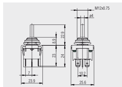
Steckanschluss 4.8 Grundtyp 1829
