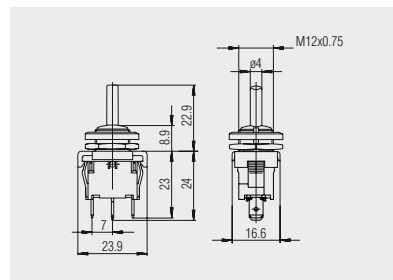
Steckanschluss 4.8 Grundtyp 1828
