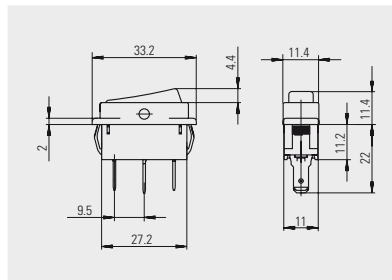
Steckanschluss 4.8 Grundtypen 1830, 1831 und 1833
