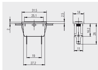
Steckanschluss 4.8 einpolige Baugröße
