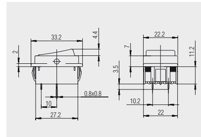
Leiterplattenanschluss Grundtypen 1832 und 1835
