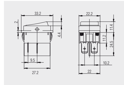
Steckanschluss 6.3 Grundtyp 1832
