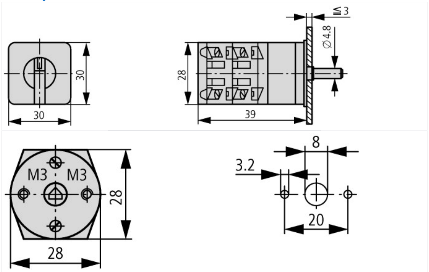
Bohrmaße Tür
