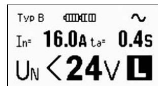
Bild 3.25 Phasenanzeige (detailliert)
