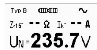
Bild 3.5 Spannungsmessung (detaillierte Darstellung).
