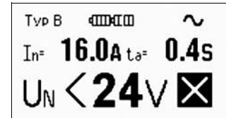
Bild 3.2 Spannung < 24 V (detaillierte Darstellung).
