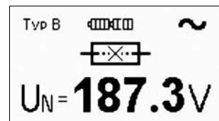
Bild 3.3 Beispiel unterbrochene Sicherung (detaillierte Darstellung).
