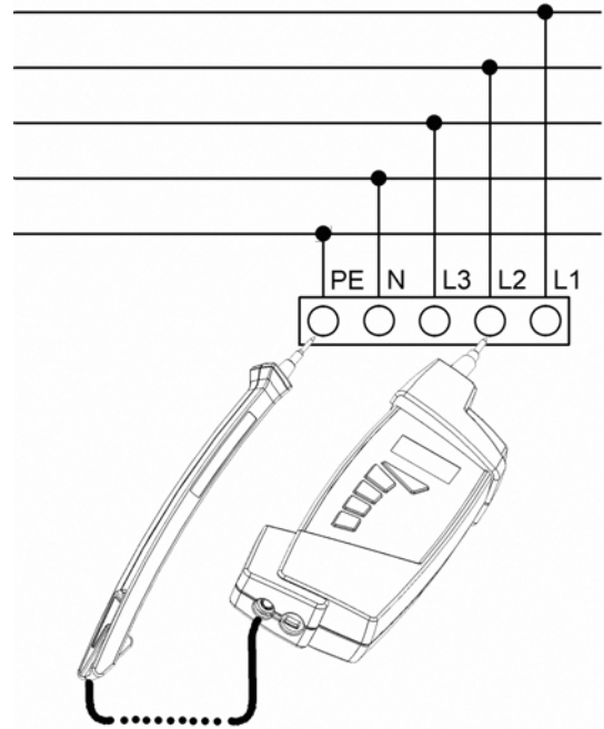
Bild 3.12 Anschlussbeispiel: Schleifenimpedanzmessung L2–PE
