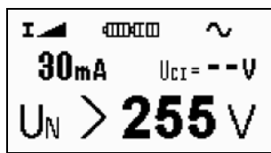
Bild 3.2 Anzeige von (Fremd-) Spannung > 255\text{ V}
