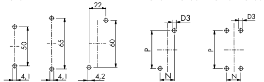
Lochbild Boden (Befestigung auf Normschiene bis KG100)
