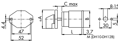
VE22/VE22-V Baugröße S0 Maß L auf der nächsten Seite
