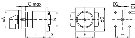
VE1 Baugröße S0, S1 Maß L auf der nächsten Seite
