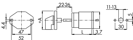
VF22/VF22-V Baugröße S0 (Nur CHR..) Maß L auf der nächsten Seite
