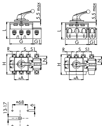
Fronteinbau 4-Loch-Befestigung
