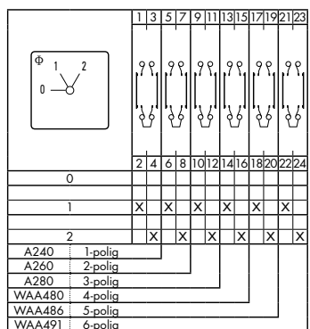
A240, A260, A280, WAA480, WAA486, WAA491
