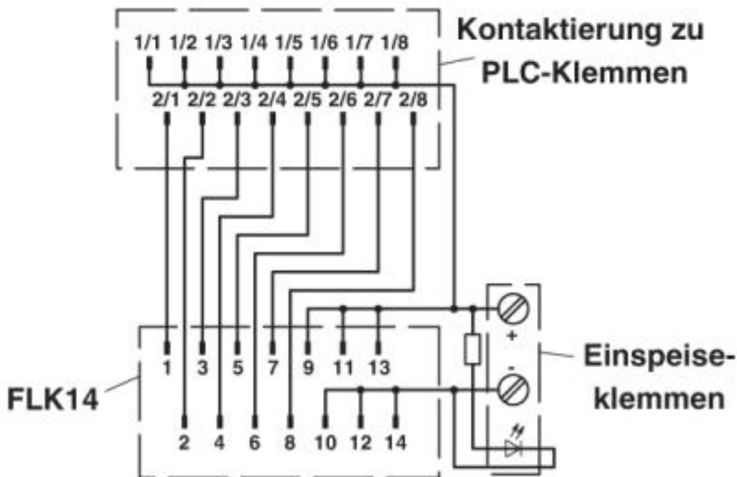
Anschlussbild PLC-V8L/FLK14/OUT/M
