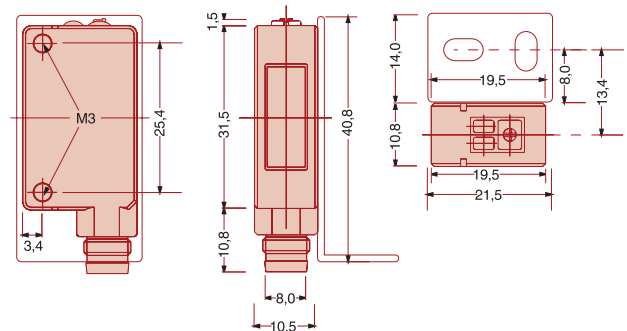
Abbildung im Maßstab 1:1. Alle Abmessungen in mm.
