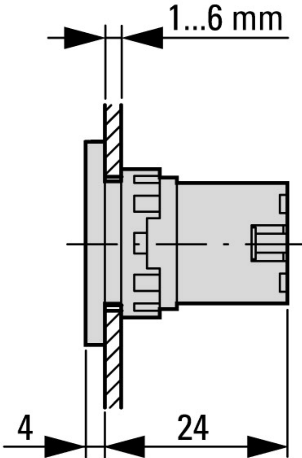
Betätigungs- und Signalisierungselemente Quadratisches Design
