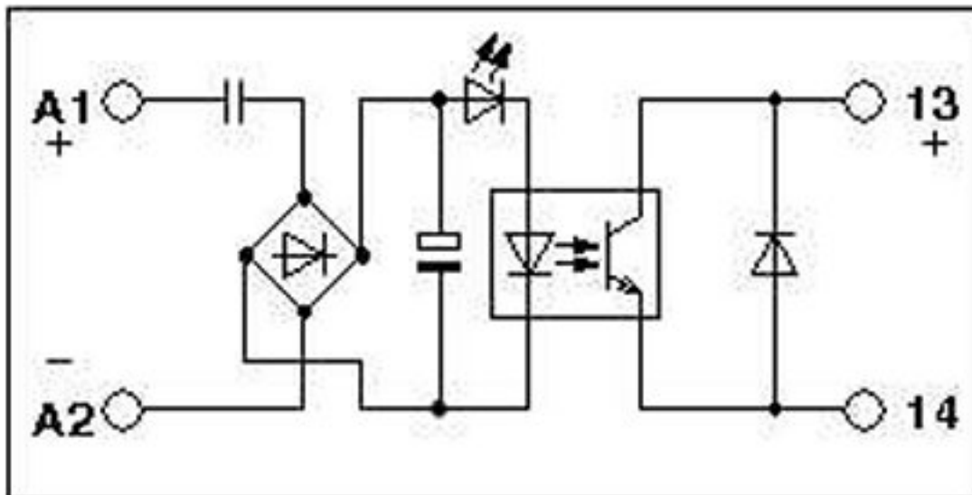
Schaltplan
