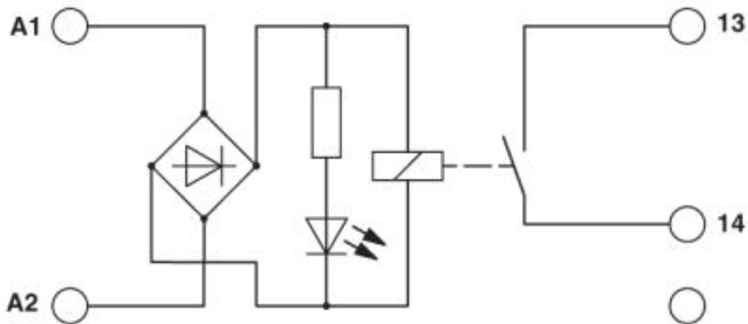
Schaltplan
