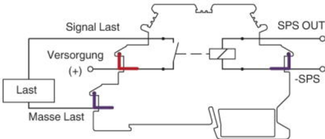
Anschlussbelegung DEK-REL-...AKT
