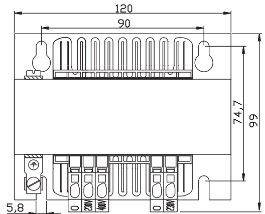
Höhe über alles / overall depth: 123mm
