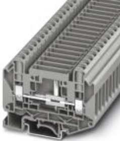
Messwandler-Trennklemme, Anschlussart: Schraubanschluss, Querschnitt: 0,2 mm 2 - 10 mm 2 , AWG: 24 - 8, Breite: 8,2 mm, Montageart: NS 35/7,5, NS 35/15, NS 32, Farbe: grau
