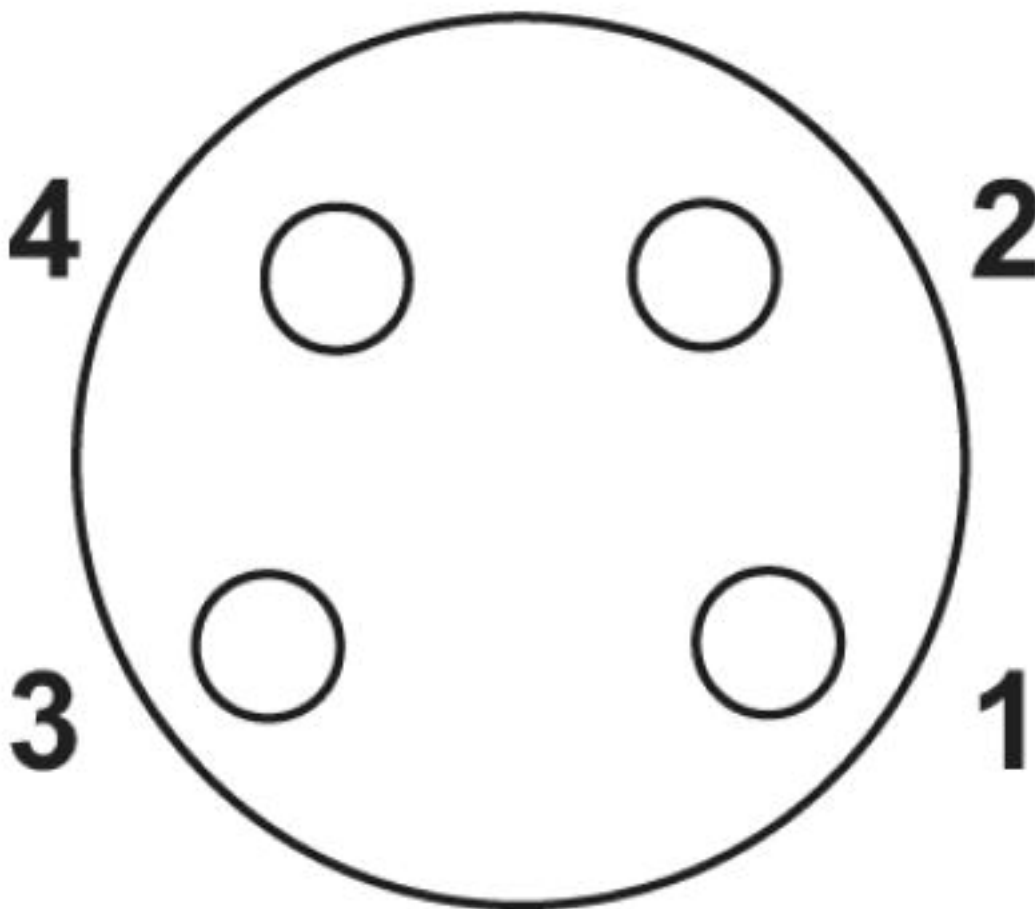
Polbild Buchse M8, 4-polig
