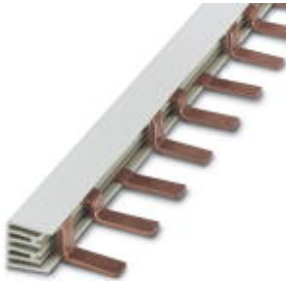
Einlegebrücke, Polzahl: 56, Farbe: grau
