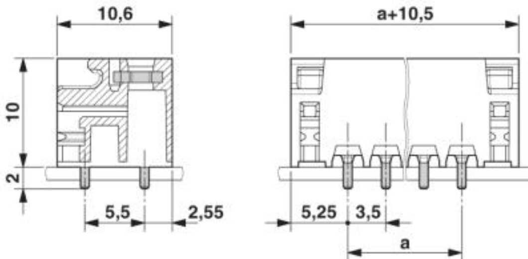
Maßzeichnung
