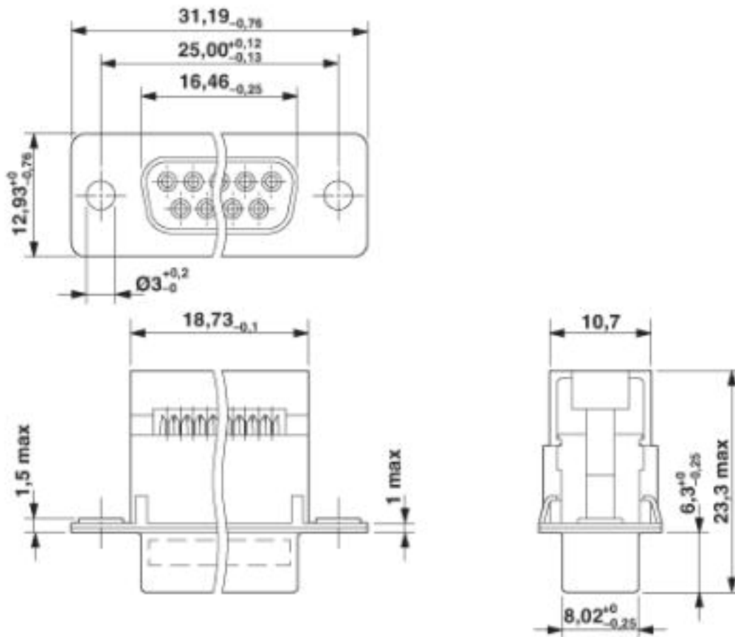
D-SUB Kontakteinsatz
