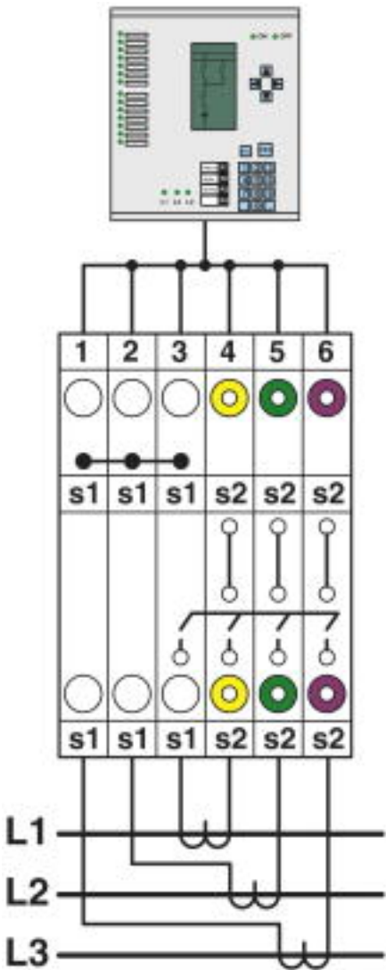
Verketteter Drei-Phasen-Stromwandlersatz
