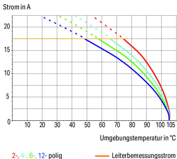
Strombelastbarkeitskurve Rastermaß 3,81 mm / Leiterquerschnitt 1,5 mm 2 „e“ In Anlehnung an: EN 60512-5-2 / Reduktionsfaktor 1
