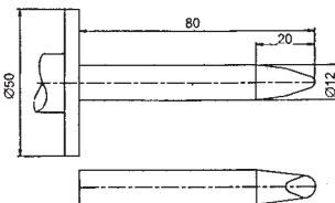
Starrer Prüffinger gemäß EN 61010-031
