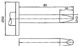
Starrer Prüffinger gemäß EN 61010-031
