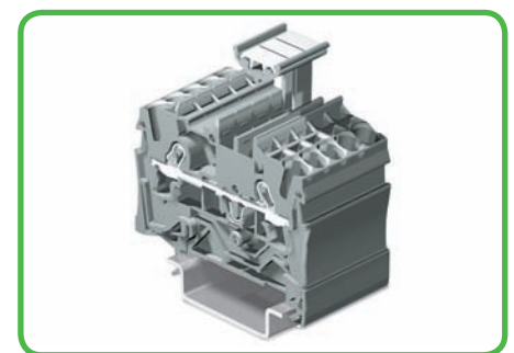
TOPJOB®S Gruppenschildträger (hier bestückt mit WMB Multibeschriftungssystem). Verwendbar für alle TOPJOB®S Reihenklemmen der Serien 2001 bis 2016
