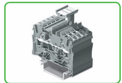
TOPJOB®S Gruppenschildträger (hier bestückt mit WMB Multibeschriftungssystem). Verwendbar für alle TOPJOB®S Reihenklemmen der Serien 2001 bis 2016
