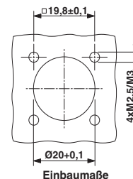
Einbaumaße
