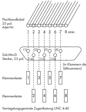
Klemmennummerierung 289-550 bis 289-554
