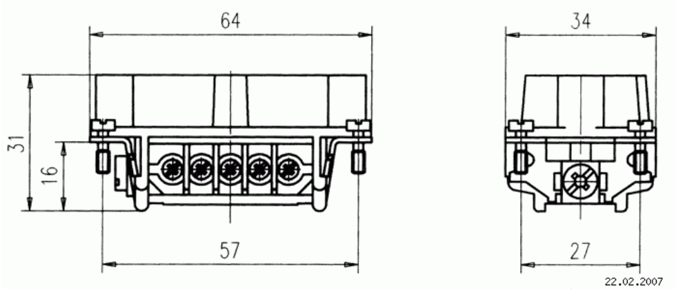
Ma zeichnung Abmessungen in mm (Inch)
