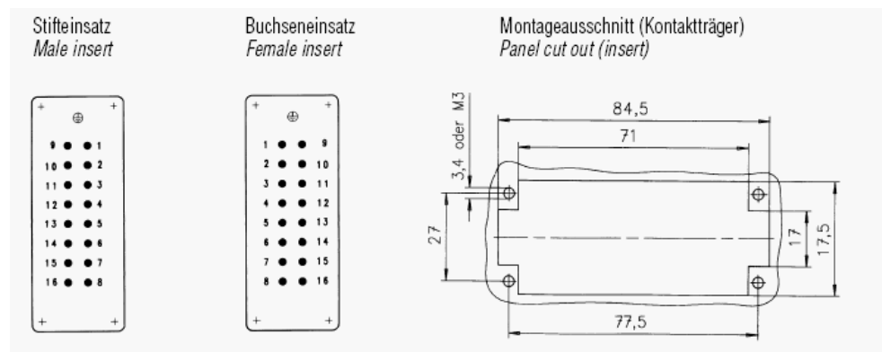
Kontaktanordnung
