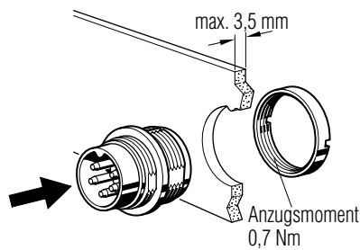
Montageausschnitt
