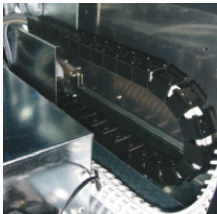
Konfektioniertes igus® System E1 an einem Pfanddrucknahmearomaten
