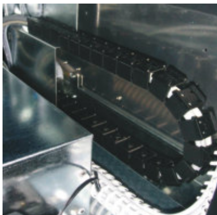
Konfektioniertes igus® System E1 an einem Pfanddrucknahemautomaten
