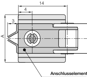
03...1Z Mitnehmer
