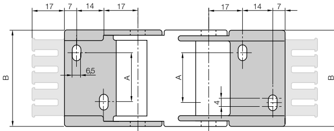
114...1P(Z) Mitnehmer
