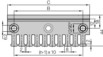
Kettenkamm einzeln
