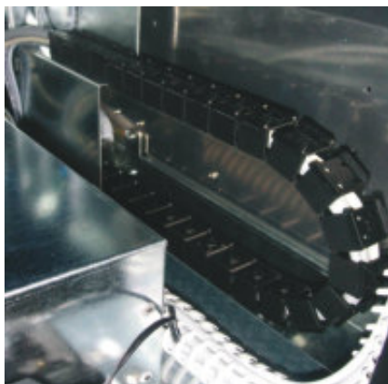
Konfektioniertes igus® System E1 an einem Pfanddrucknahmeautomaten
