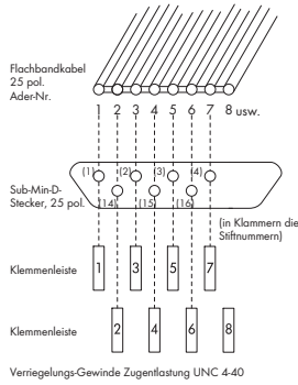
Klemmennummerierung 289-550 bis 289-554
