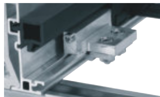
Prinzipzeichnung: Anzahl der zu montierenden Montagesets Basic = Anzahl der Rinneinstücke + 1
