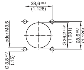
Montageausschnitt
